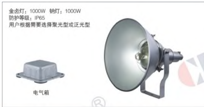
CNT9150A 防震高亮度投光灯
